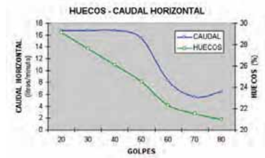
Figura 6: Gráfico de huecos y caudal horizontal con las diferentes energías aplicadas.
