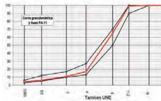
Figura 3: Gráfico de la curva granulométrica y huso PA 11.
